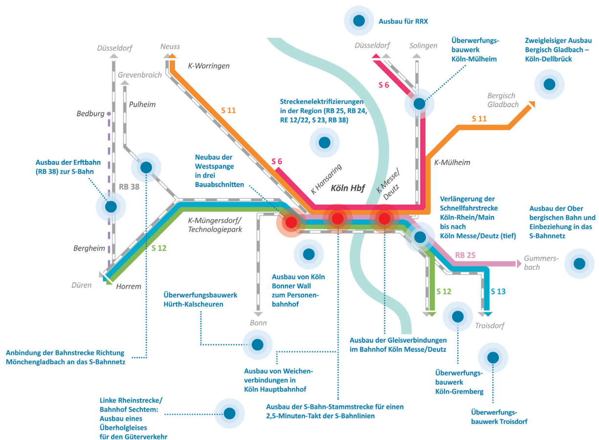
Abb.2: Maßnahmen im Knoten Köln
