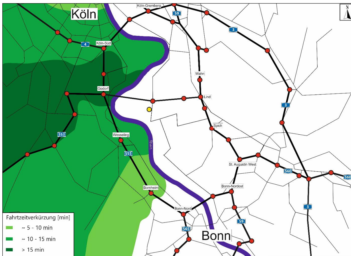
Abbildung 29: Zeiterparnisse im Prognose-Planfall 1 2030 gegenüber dem Prognose-Bezugsfall Rheinspange 2030 für den Ortsteil Ranzel der Stadt Niederkassel
