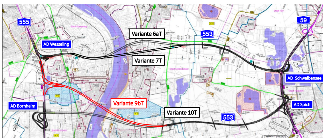
Abbildung 1: Lage des Tunnels (Quelle: Autobahn GmbH des Bundes)
